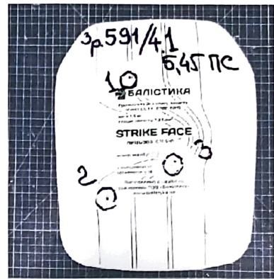
Фото зразка № 591/4.1 після випробувань
