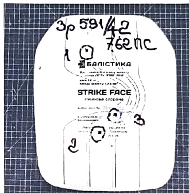
Фото зразка № 591/4.2 після випробувань
